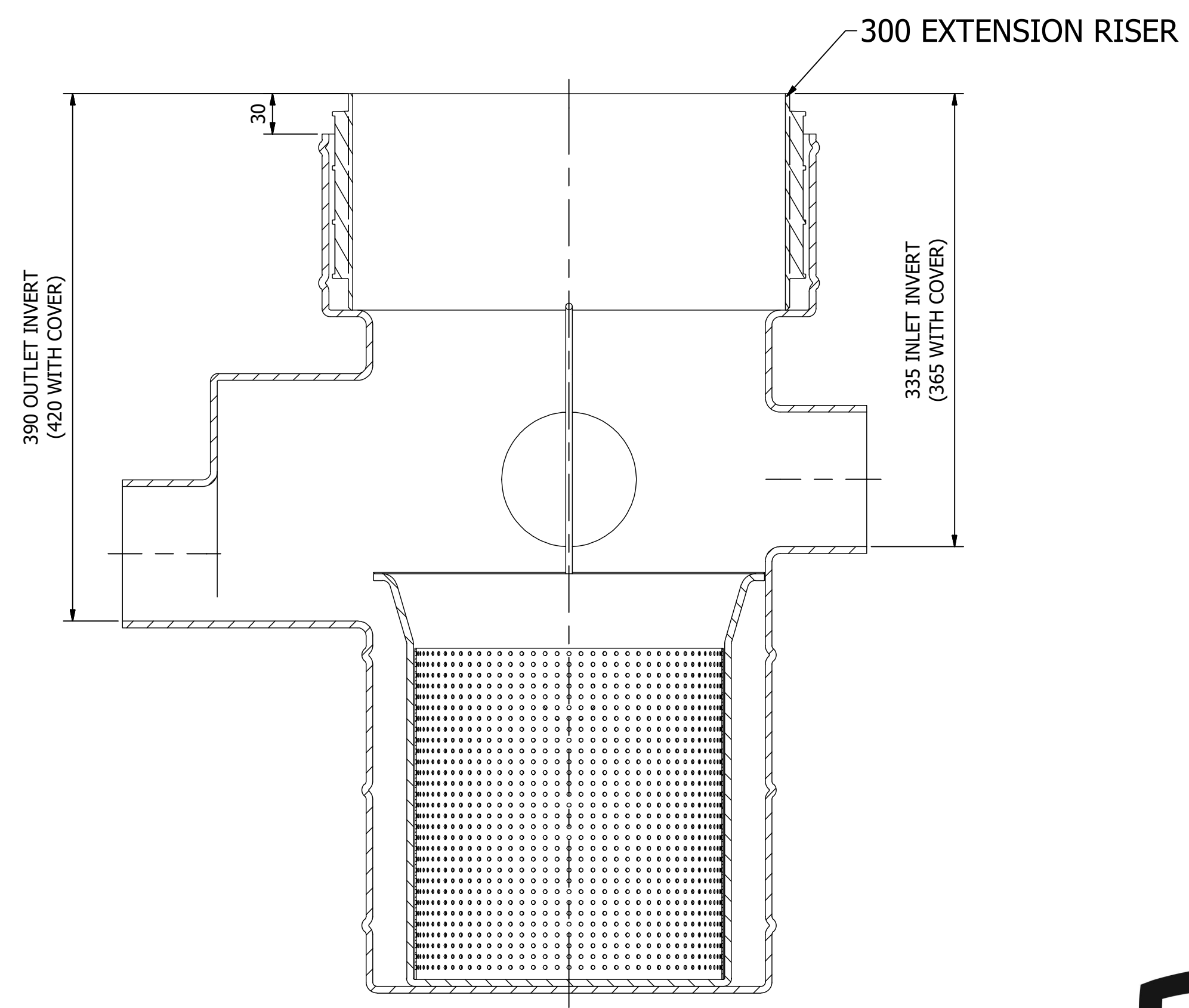
SECTION A-A SCALE 1:3.333
